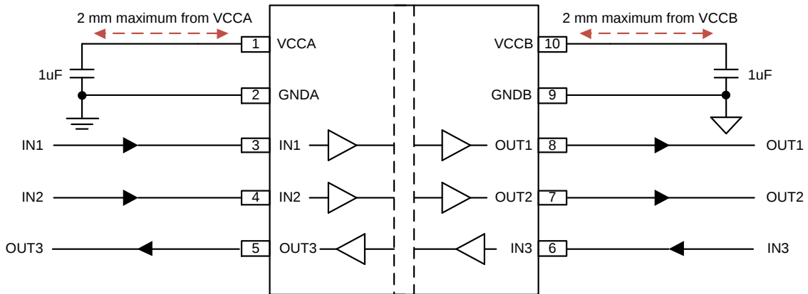
图 12-1. UMISO7331U 典型应用
