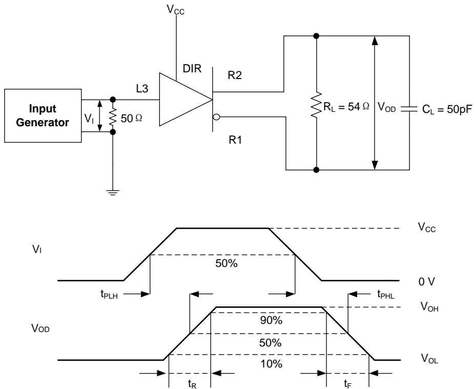
图 9-3. RS-485 驱动器差分输出上升和下降时间及传播延迟的测量
