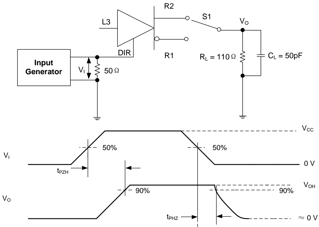
图 9-4. 具有高电平有效输出和下拉负载的 RS-485 驱动器使能和禁用时间测量
