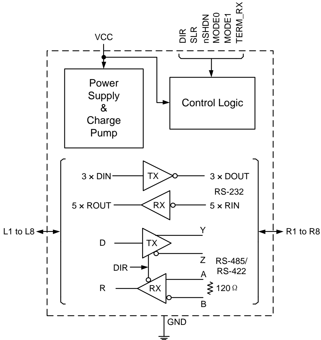
图 10-1. UM3035B 框图
