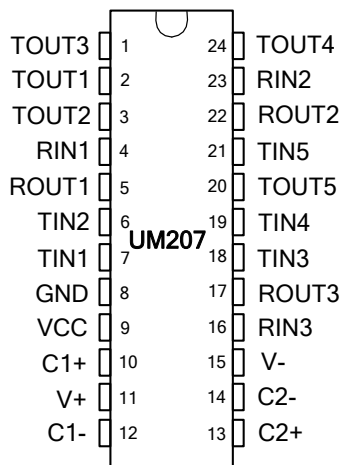
SOP24/SSOP24/TSSOP24
