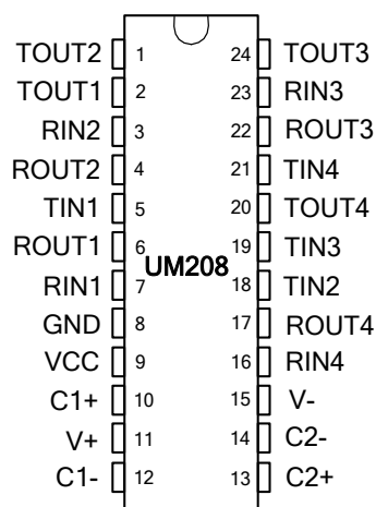
SOP24/SSOP24/TSSOP24
