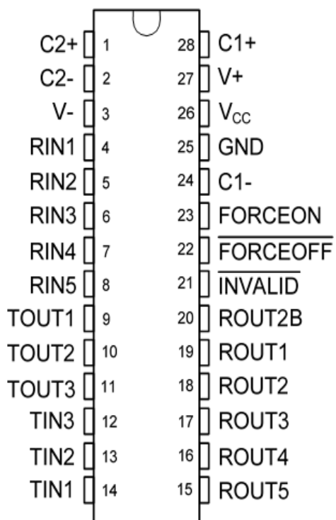
SSOP28/TSSOP28/SOP28
